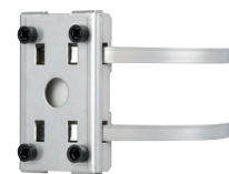
ポールアタッチメント (BP-02) 適合ポール径: φ40mm~φ140mm
